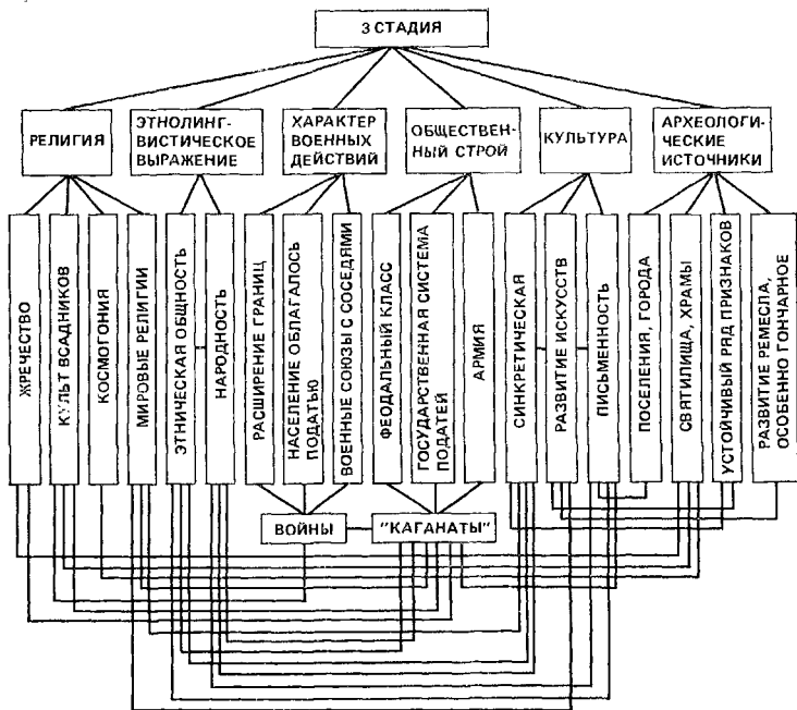
Рис. 3. Схема взаимосвязей признаков на третьей стадии кочевания (модель 3)
