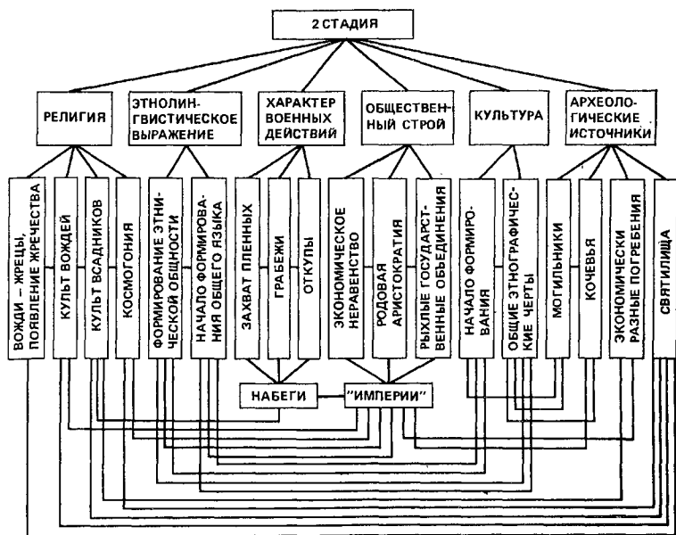
Рис. 2. Схема взаимосвязей признаков на второй стадии кочевания (модель 2)
